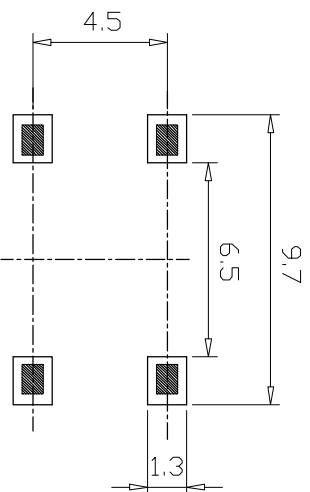
P. C. B. Layerrout di agram
